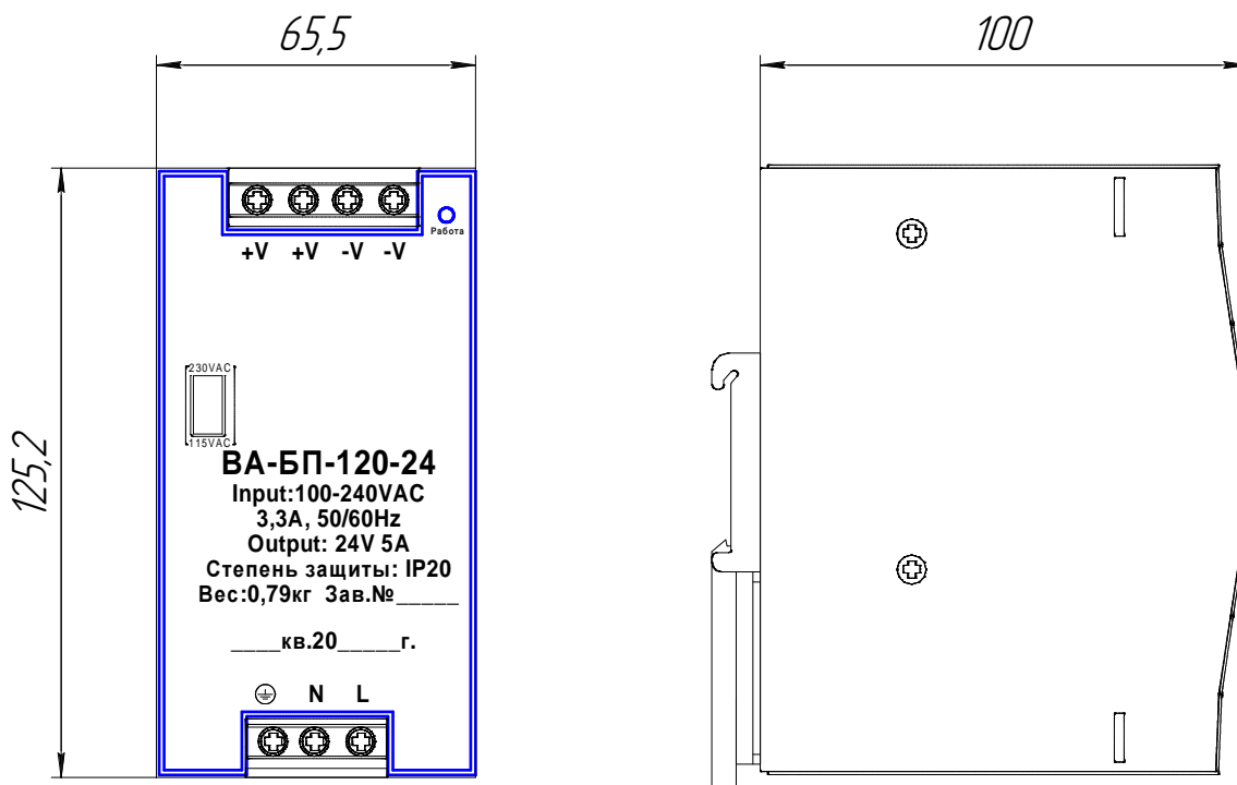
Габаритно-установочные размеры ВА-БП-120-24
