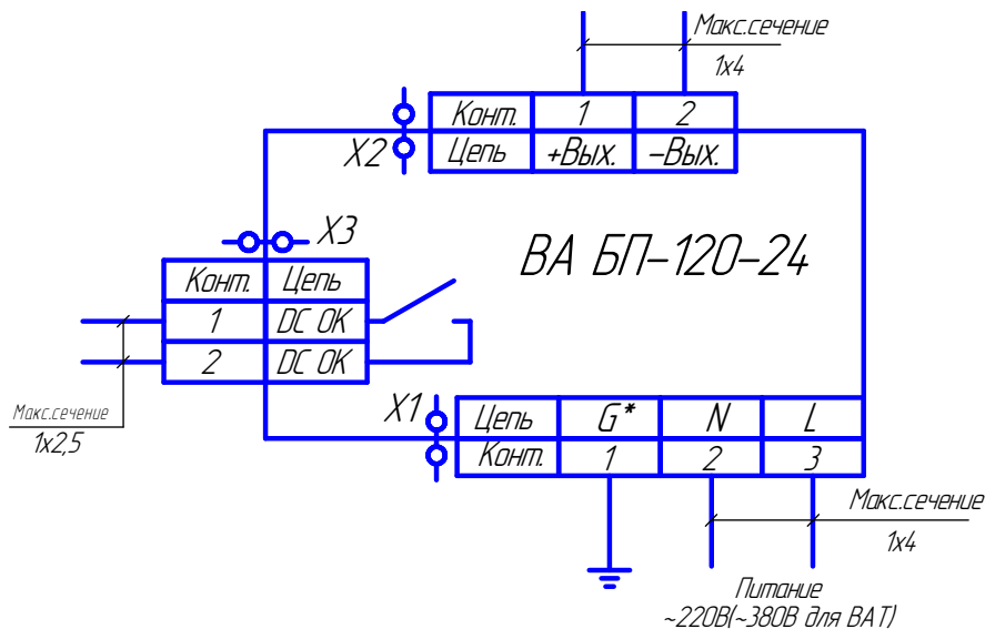
Схема внешних подключений ВА-БП-120-24
