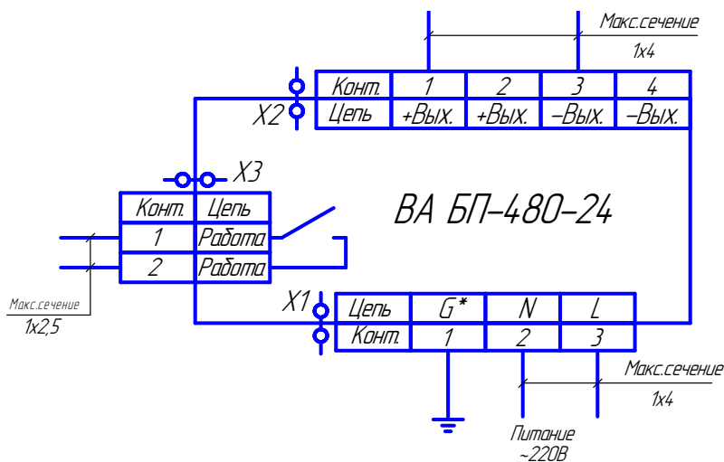
Схема внешних подключений ВА-БП-480-24
