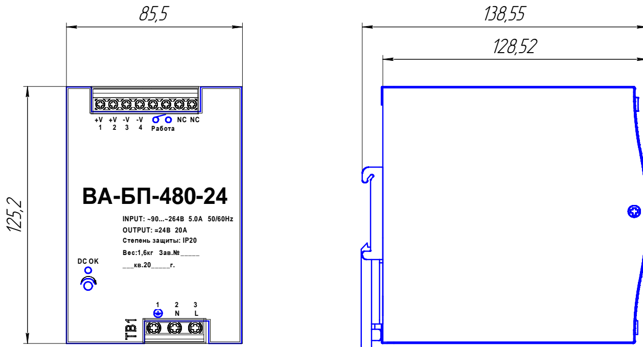
Габаритно-установочные размеры ВА-БП-480-24
