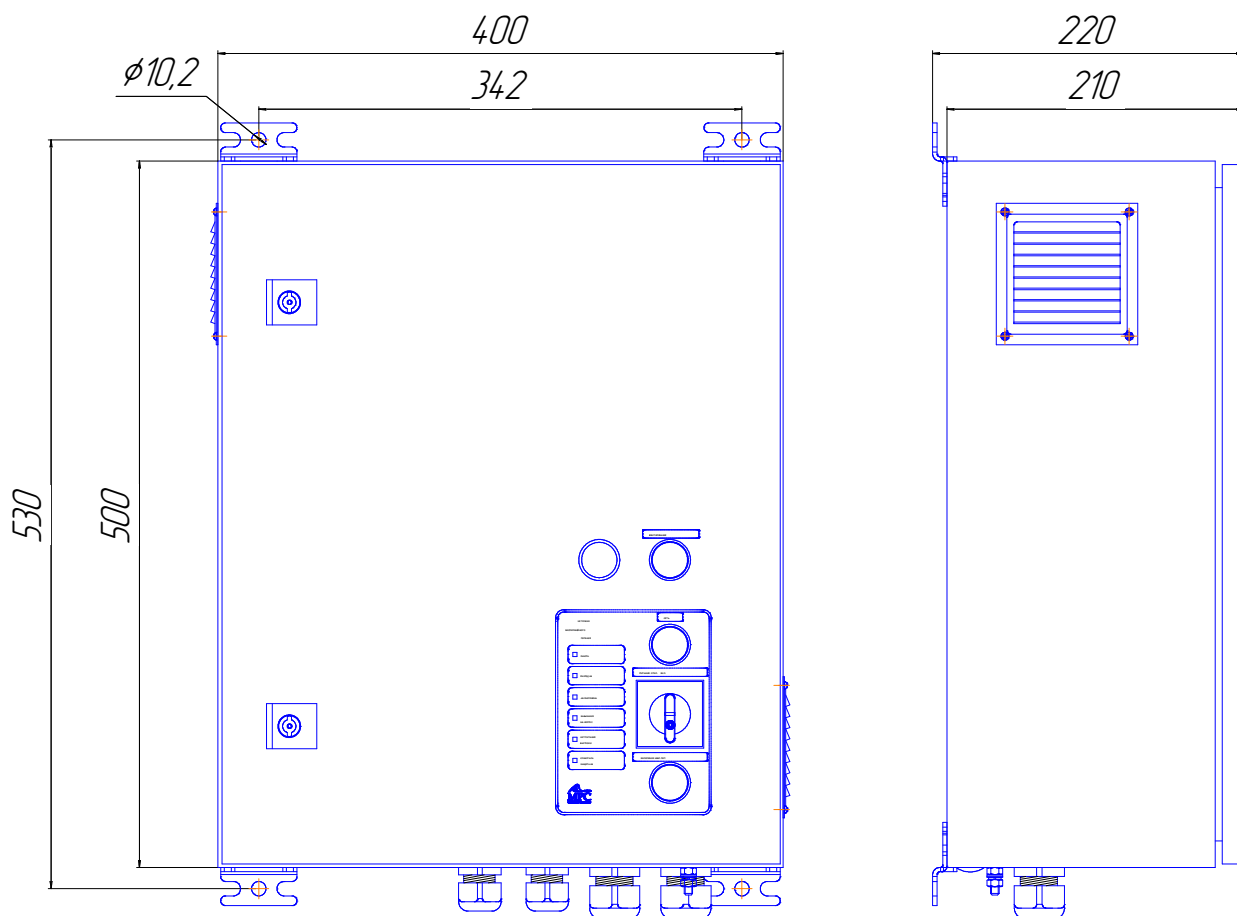
Прибор ВА ИБП-220/24-17-10 Габаритно установочные размеры
