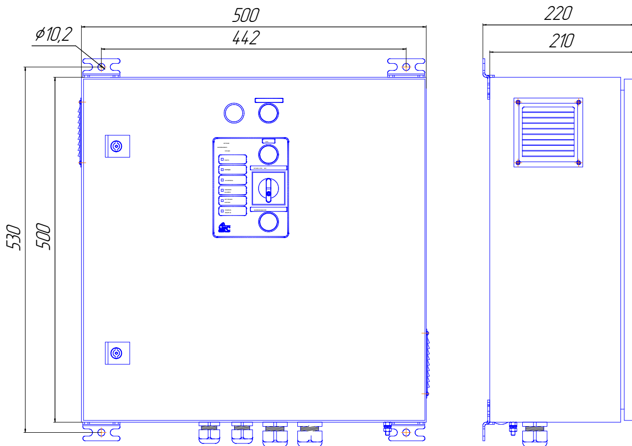
Прибор ВА ИБП-220/24-40-10 Габаритно установочные размеры
