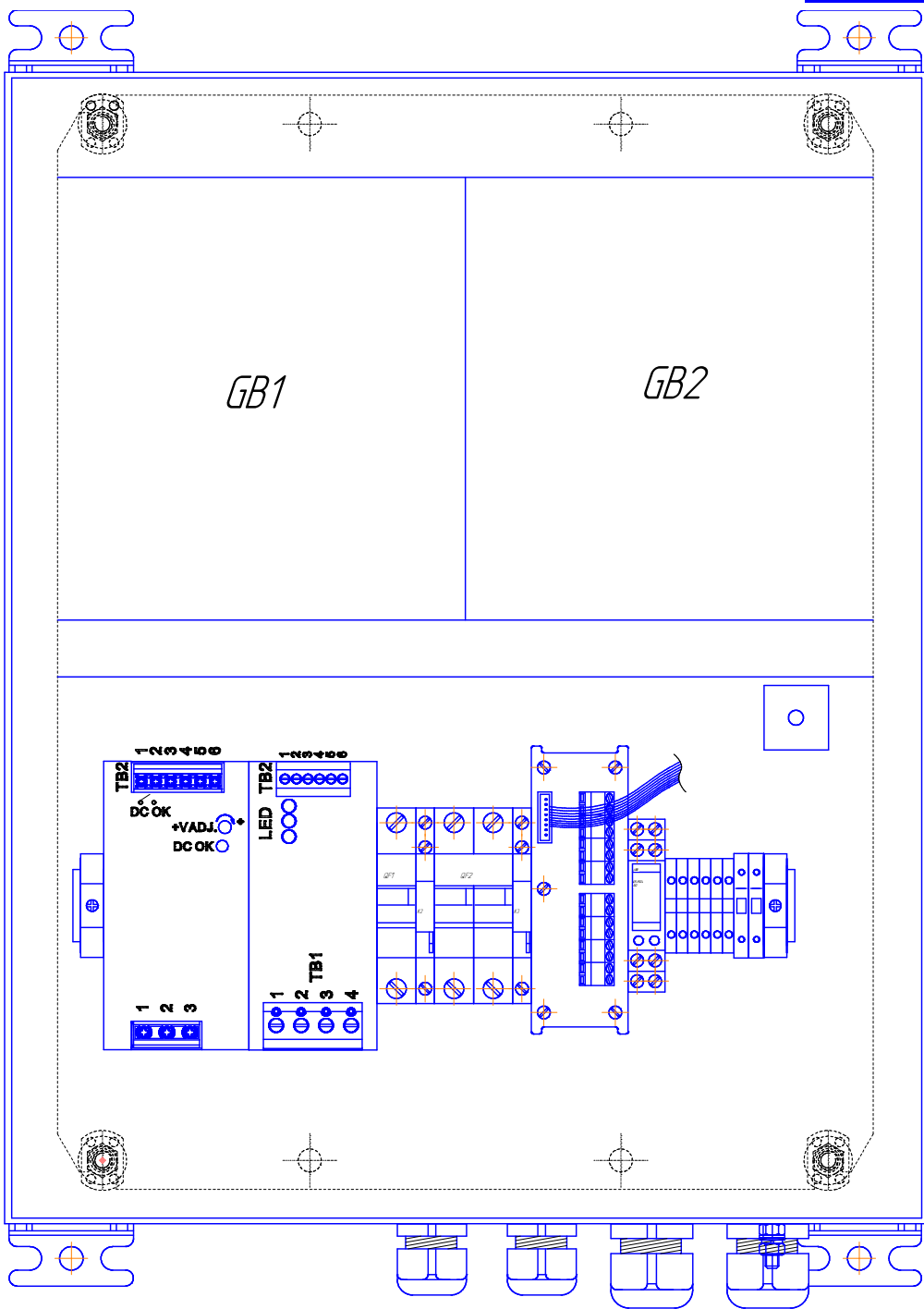
Прибор ВА ИБП-220/24-40-10 Вид щита с открытой дверцей (расположение элементов внутри щита может отличаться от представленного)
