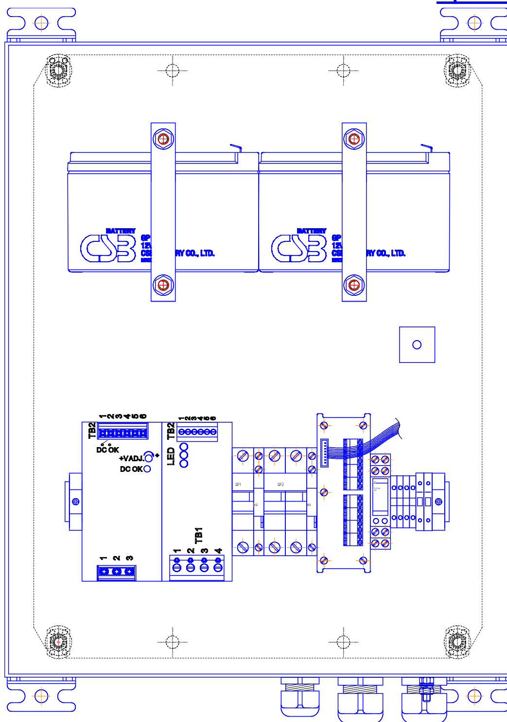
Прибор ИБП-220/24-12 Вид щита с открытой дверцей
