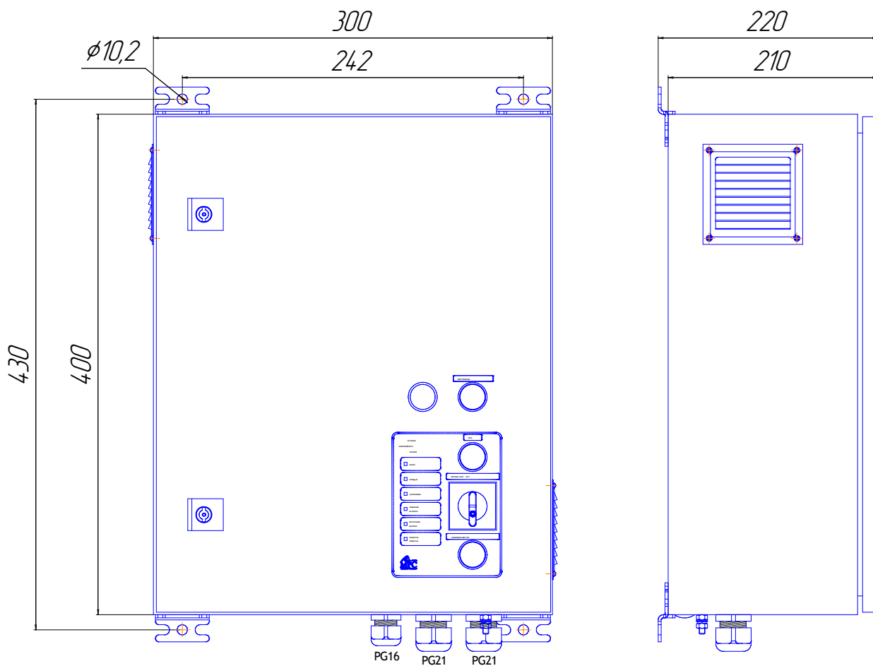
Прибор ИБП-220/24-12 Габаритно установочные размеры
