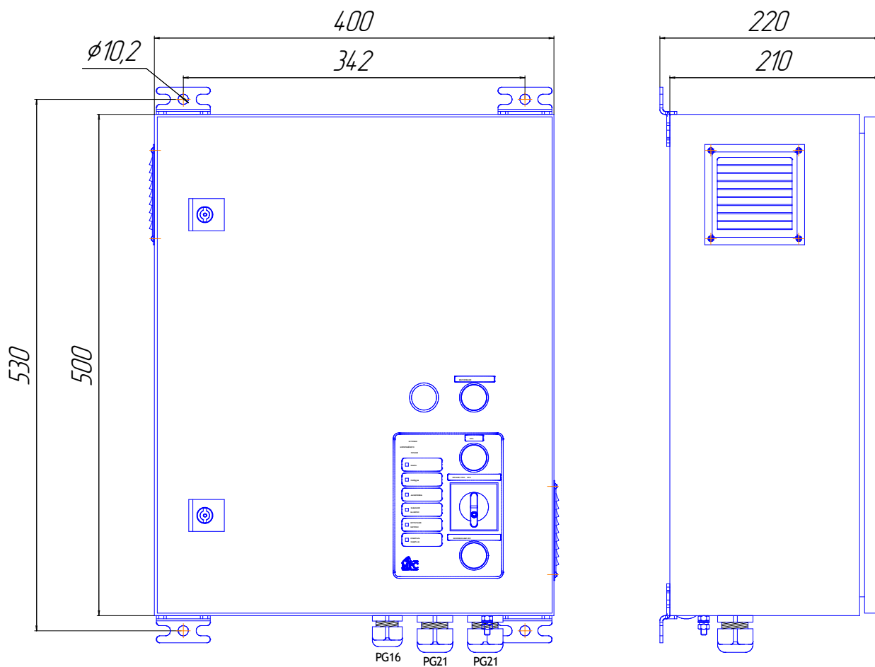
Прибор ИБП-220/24-26 Габаритно установочные размеры
