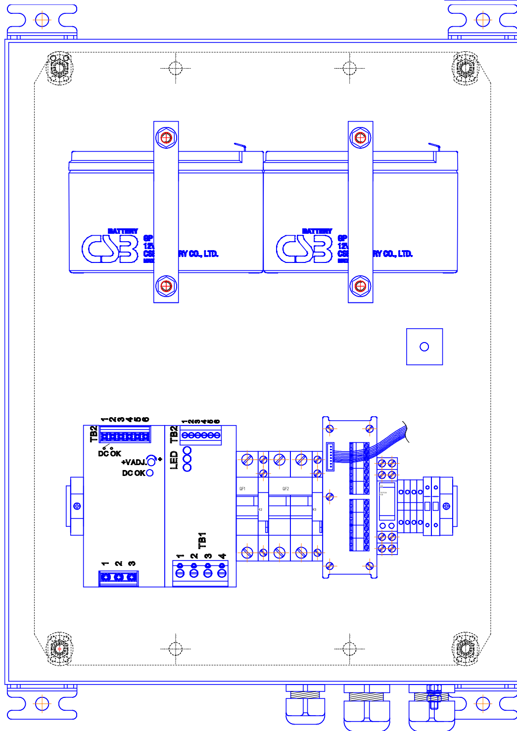
Прибор ИБП-220/24-26 Вид щита с открытой дверцей
