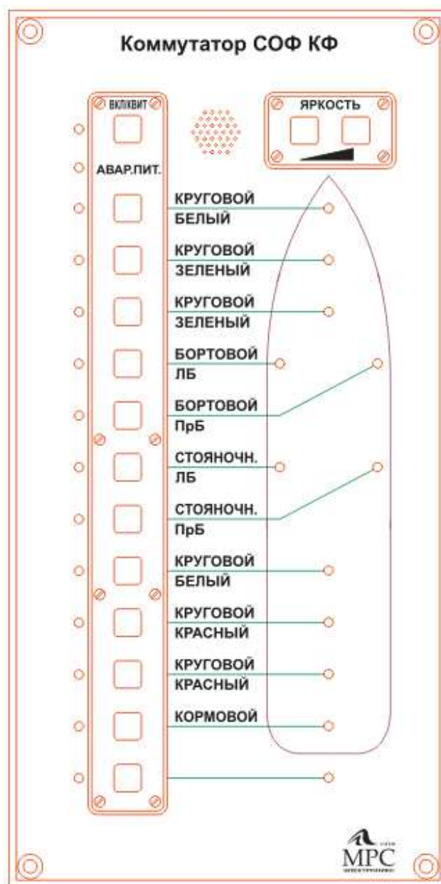
Внешний вид лицевой панели КФ-24-12
