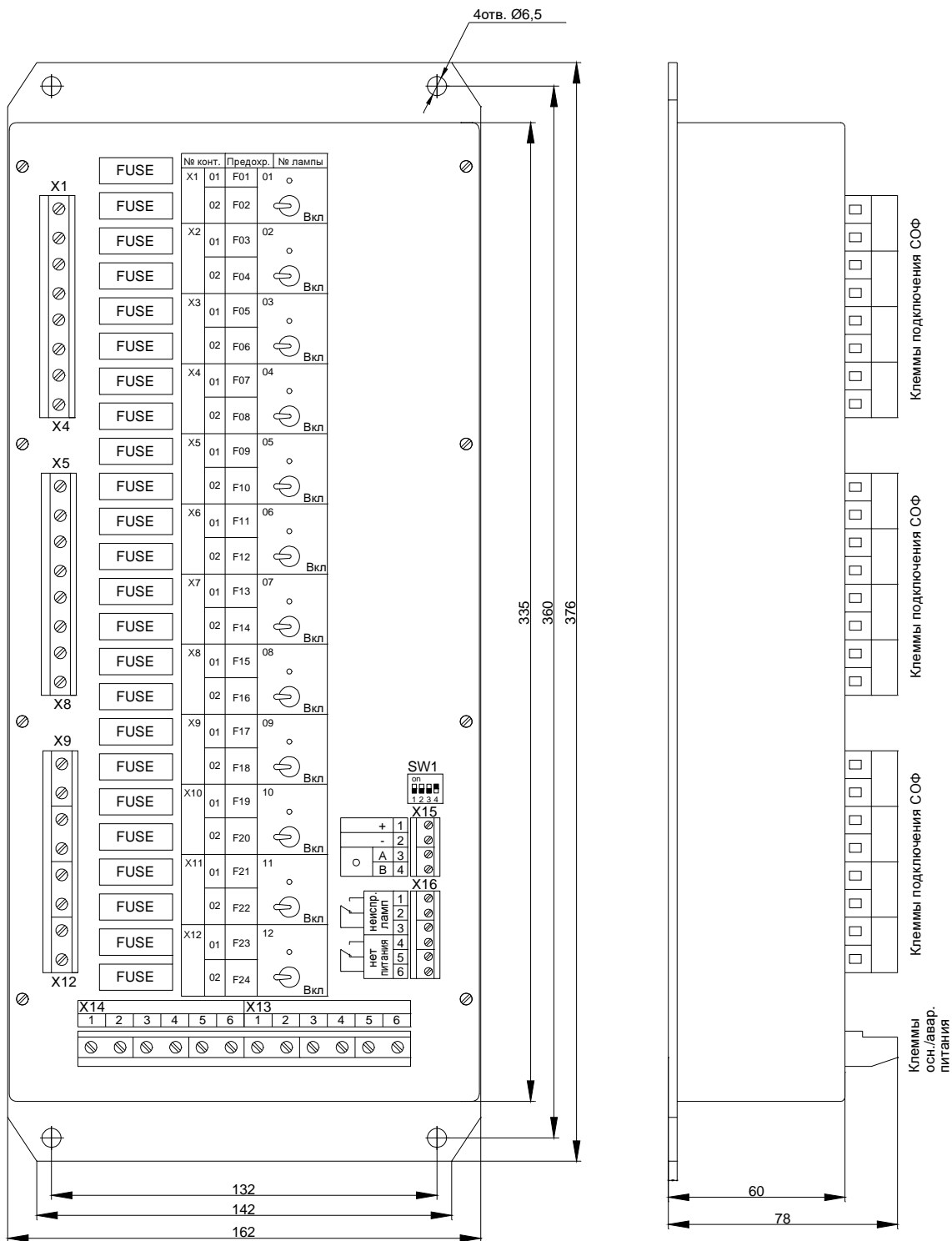
Блок силовой БС КФ-24-12
