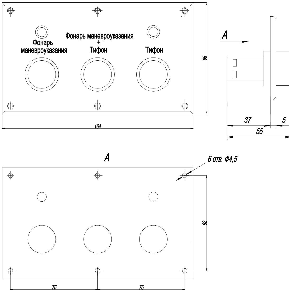
Пост кнопочный КП Габаритно-установочный размер
