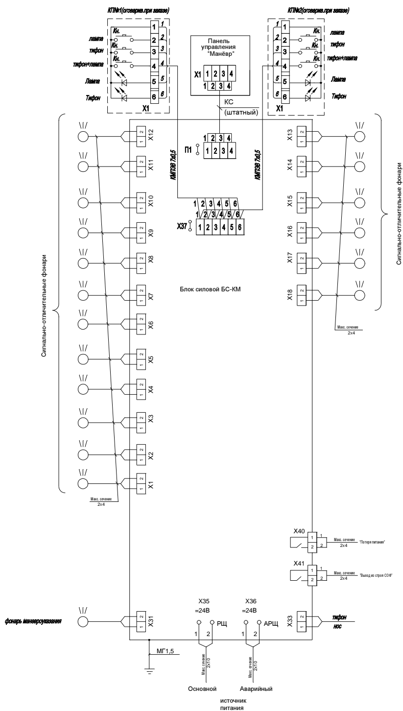
Схема электрическая подключений комплекта "Маневр"
