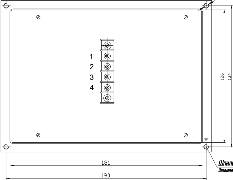
Вид сзади
