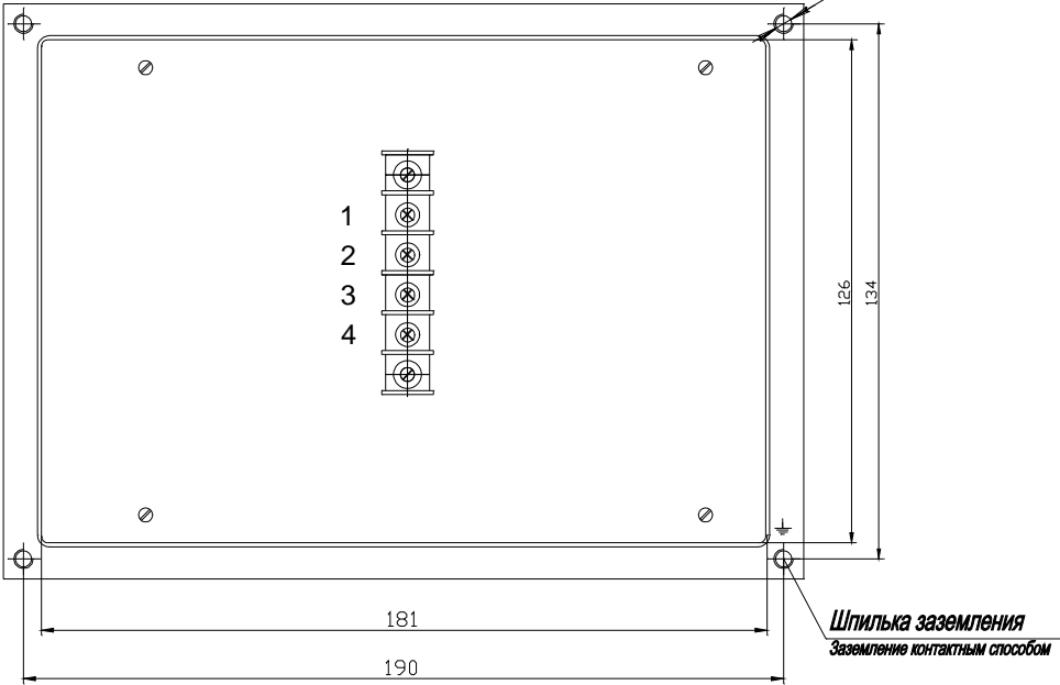
Вид сзади
