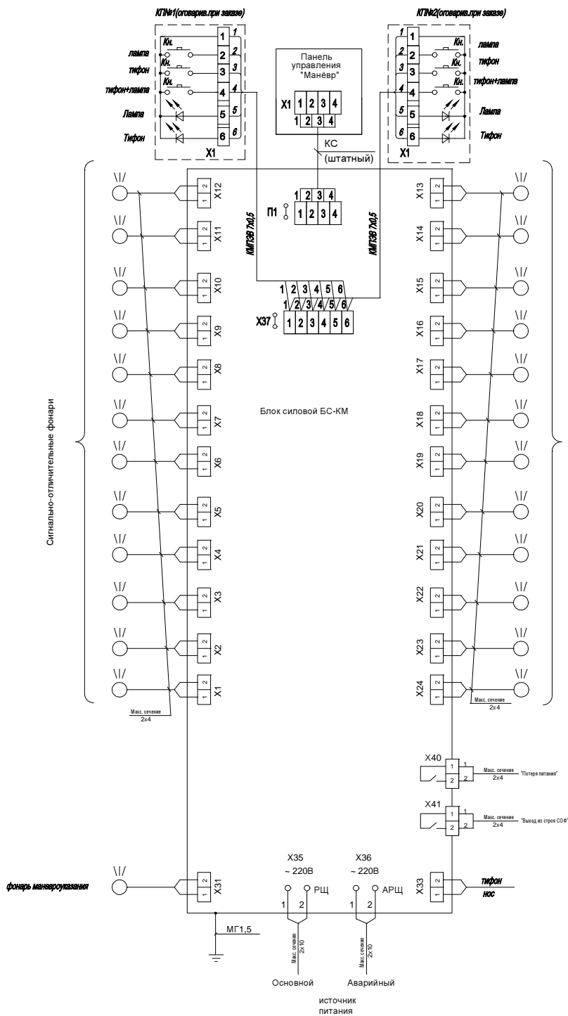
Схема электрическая подключений комплекта “Манёвр”
