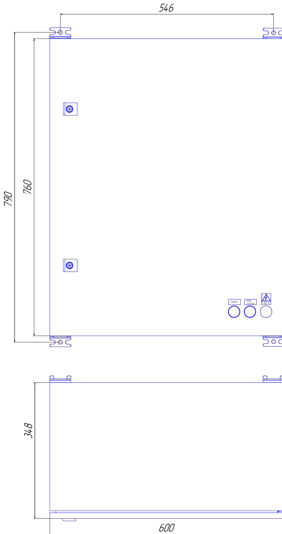
Телефонная станция КТ-96 Габаритный чертёж
