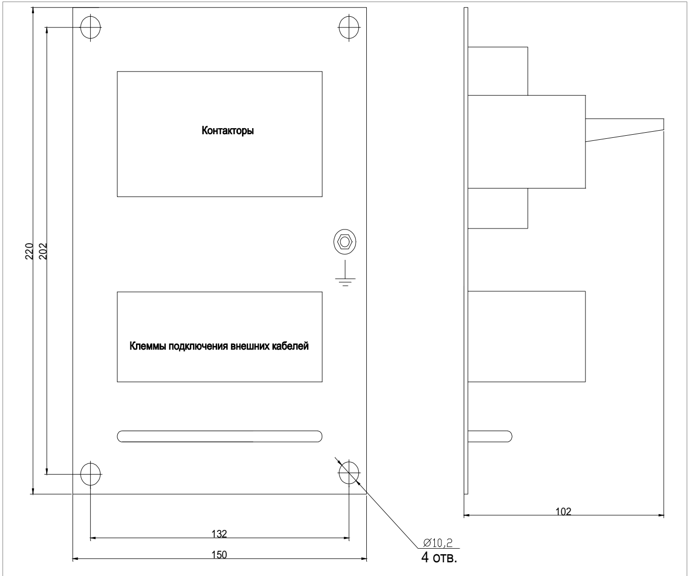
Блок БКП-24 Габаритный чертёж
