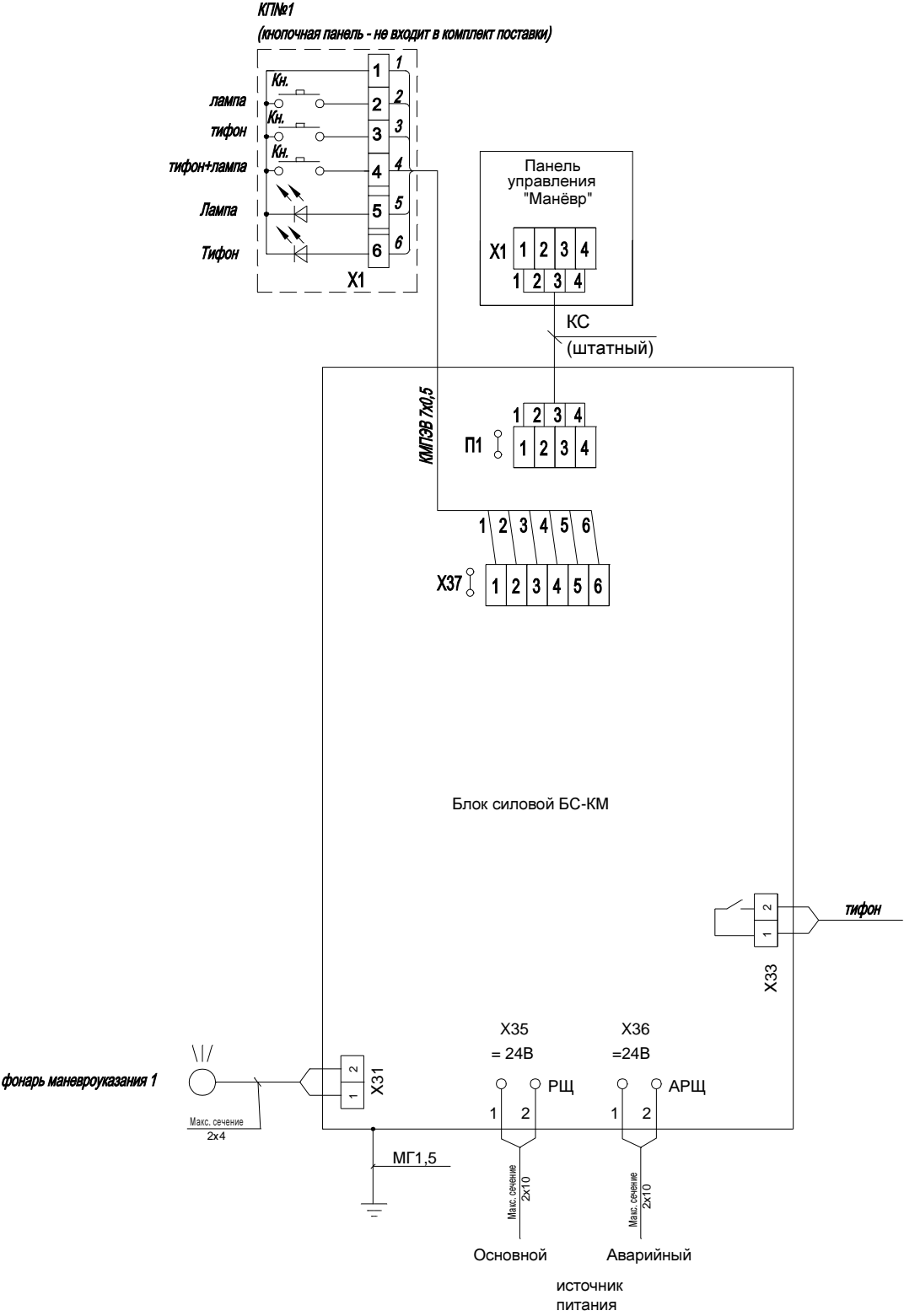
Схема электрическая подключений прибора “Маневр”
