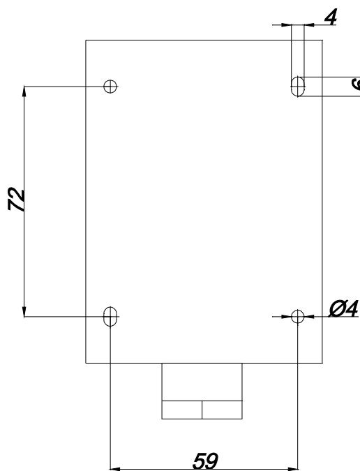
Вид сзади
