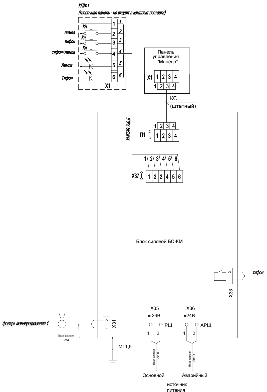
Схема электрическая подключений прибора "Маневр"
