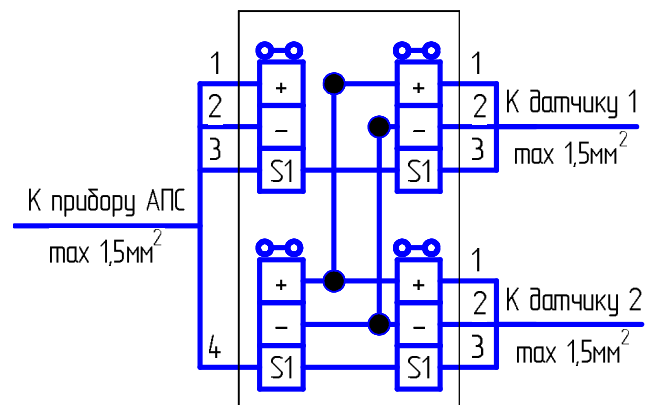
Коробка соединительная СК4 (S2) Схема принципиальная
