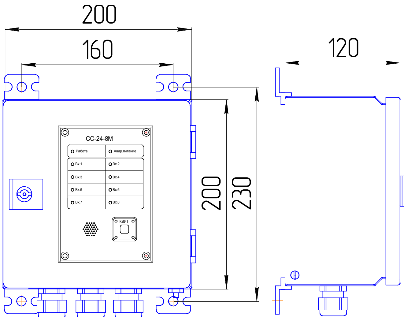
Панель СС-24-8МЩ IP44 Габаритно установочные размеры
