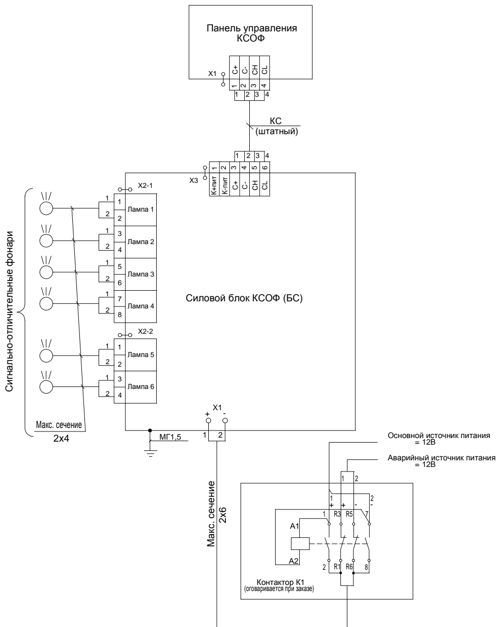
Схема соединений
