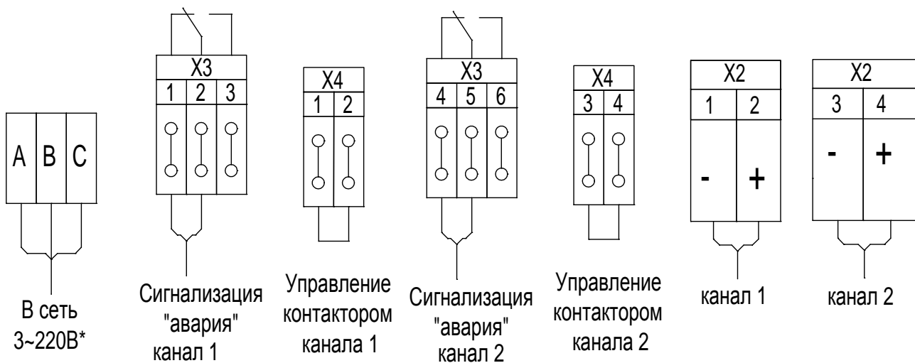
Подключение внешних кабелей
