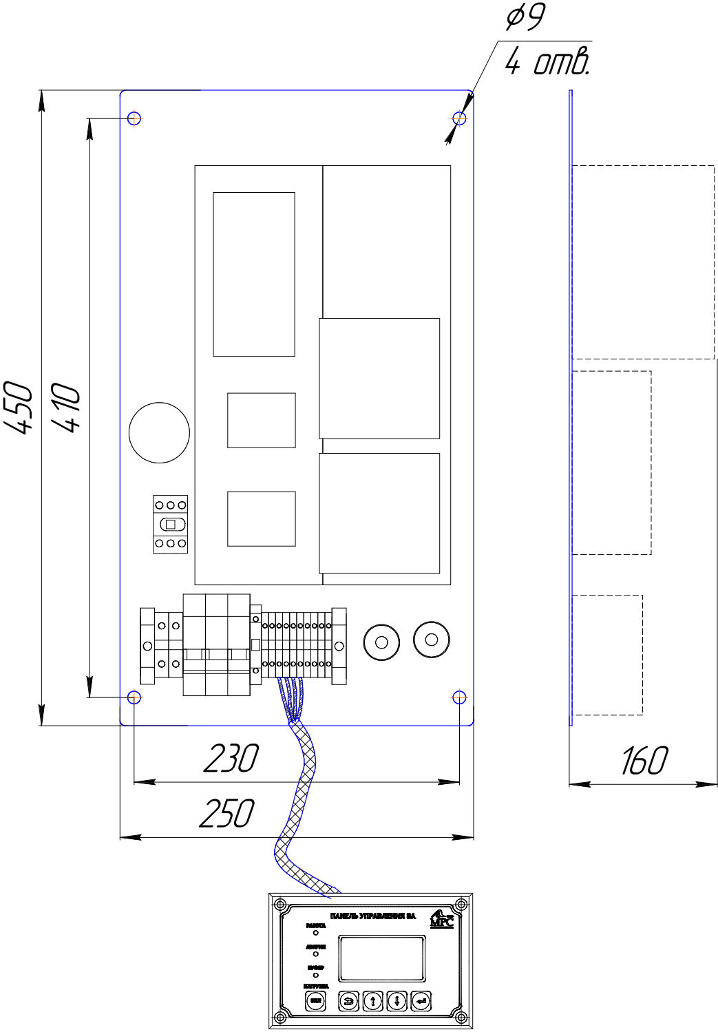
Агрегат ВА2450 IP20
