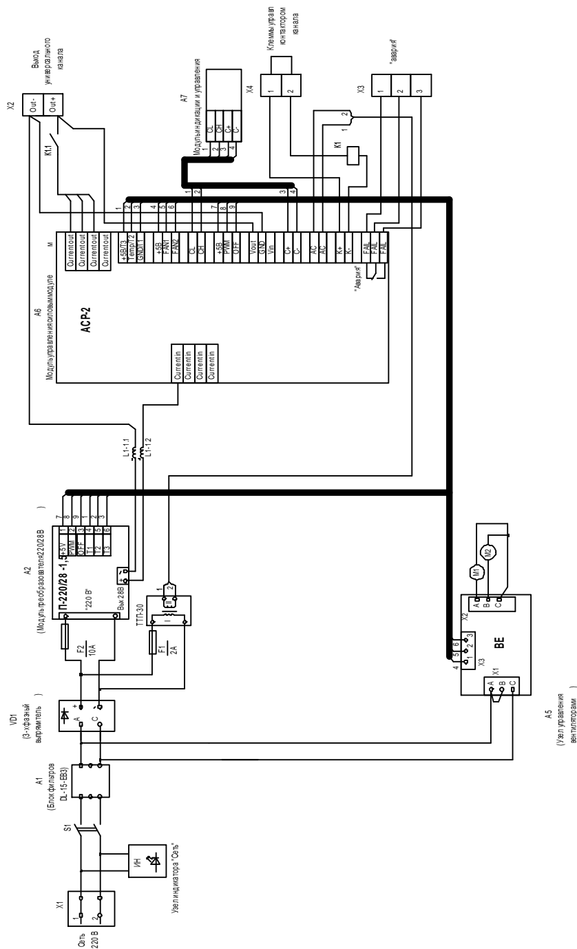
Агрегат ВА2450 Схема электрическая принципиальная
