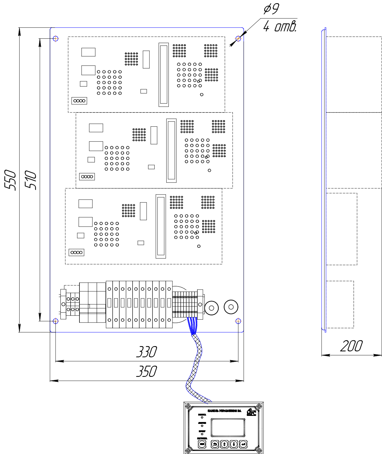
Агрегат ВАТ24100 IP20 Габаритно-установочные размеры
