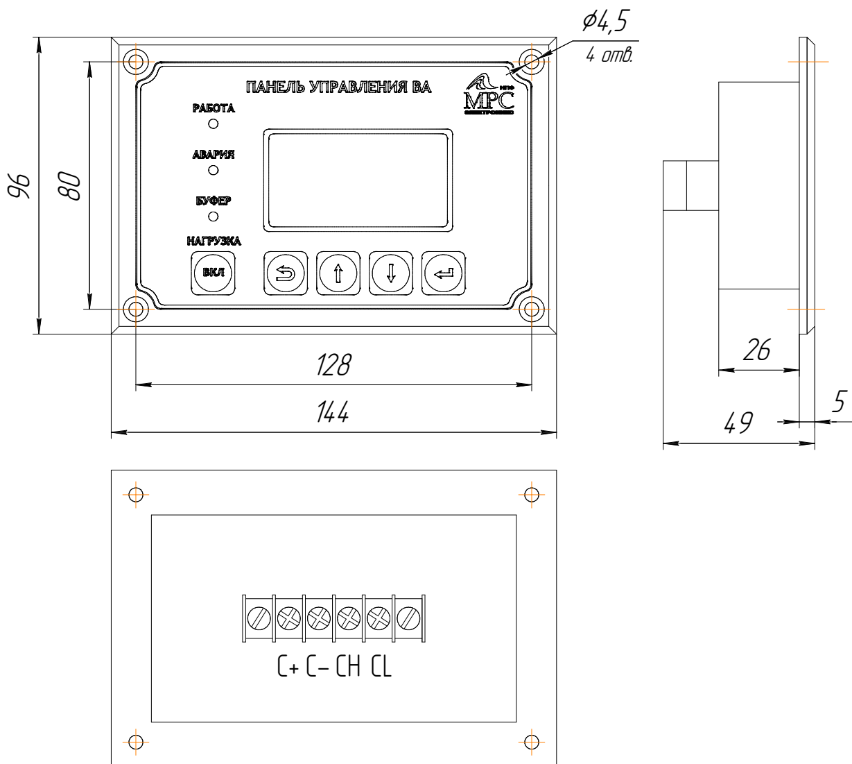
выносная панель ПУВА Габаритно-установочные размеры
