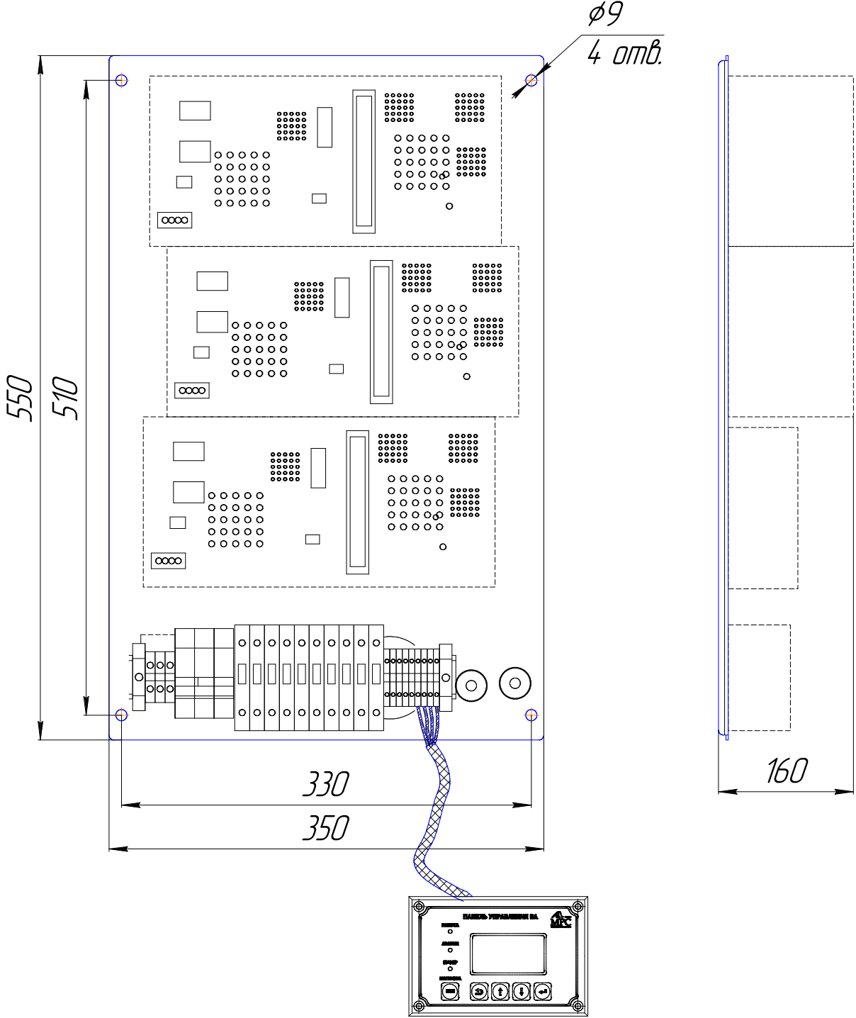
Агрегат ВА24150 IP20 с выносной панелью ПУВА Габаритно-установочные размеры
