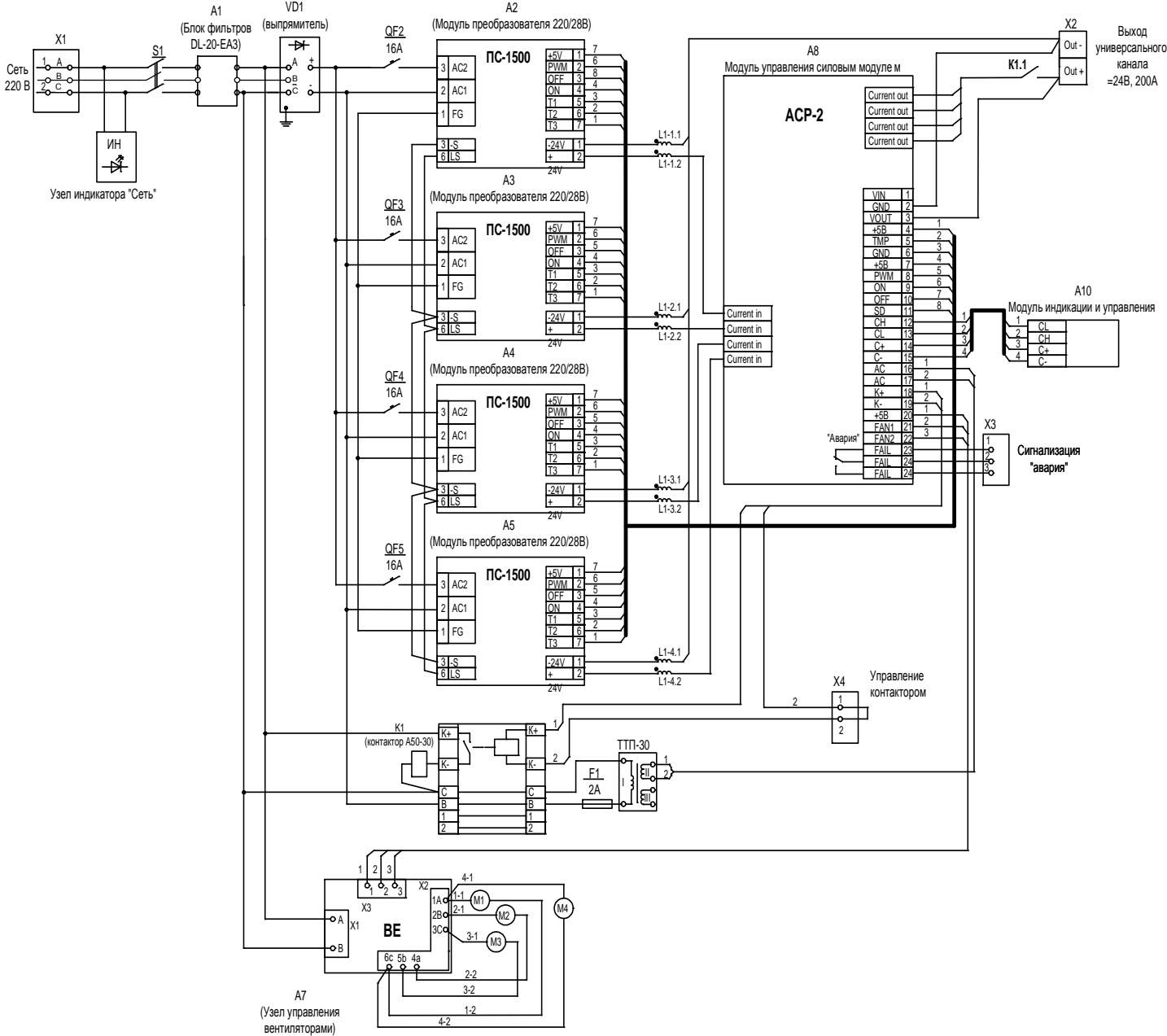
Агрегат ВА24150 IP20 с выносной панелью ПУВА Схема электрическая принципиальная
