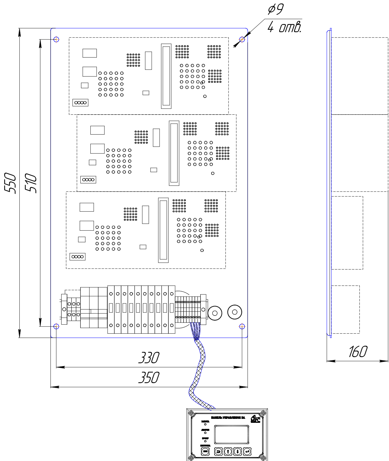
Агрегат ВАТ24200 IP20 Габаритно-установочные размеры
