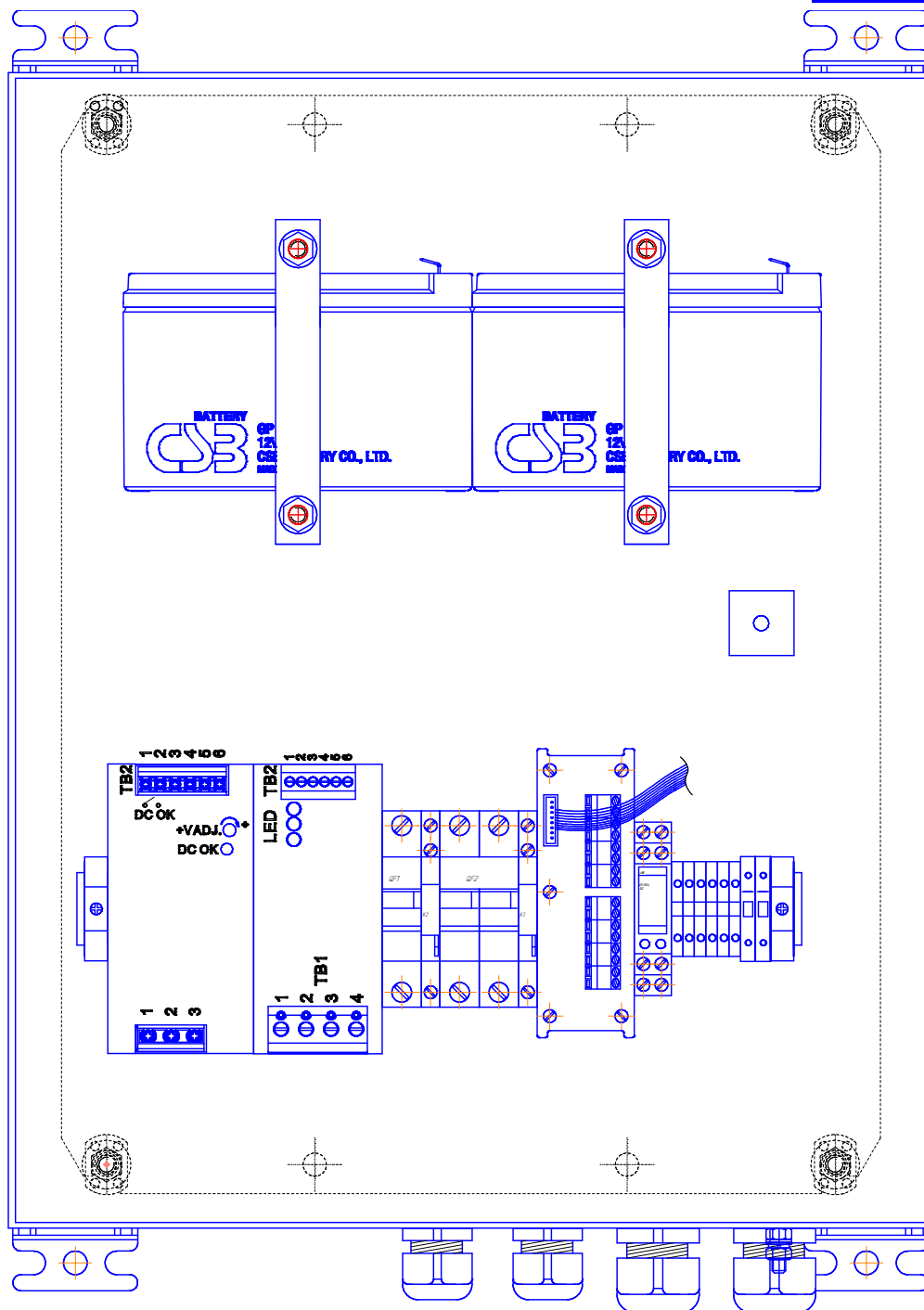
Прибор ВА ИБП-220/24-7,2-5 Вид щита с открытой дверцей (расположение внутренних элементов внутри щита может отличаться от представленного)
