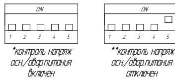
Варианты выставление DIP перкл. на силовом блоке БС КМ контроль питания:
