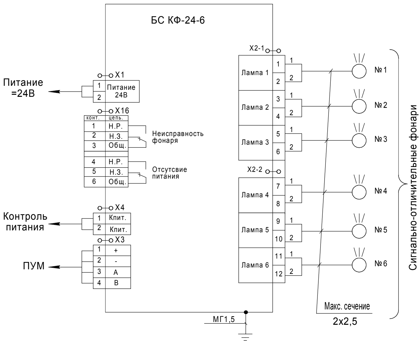
Блок силовой BS KF-24-6 Схема электрическая подключений
