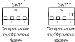
Варианты выставление DIP переключ. на силовом блоке BS KF-6 контроль питания:
