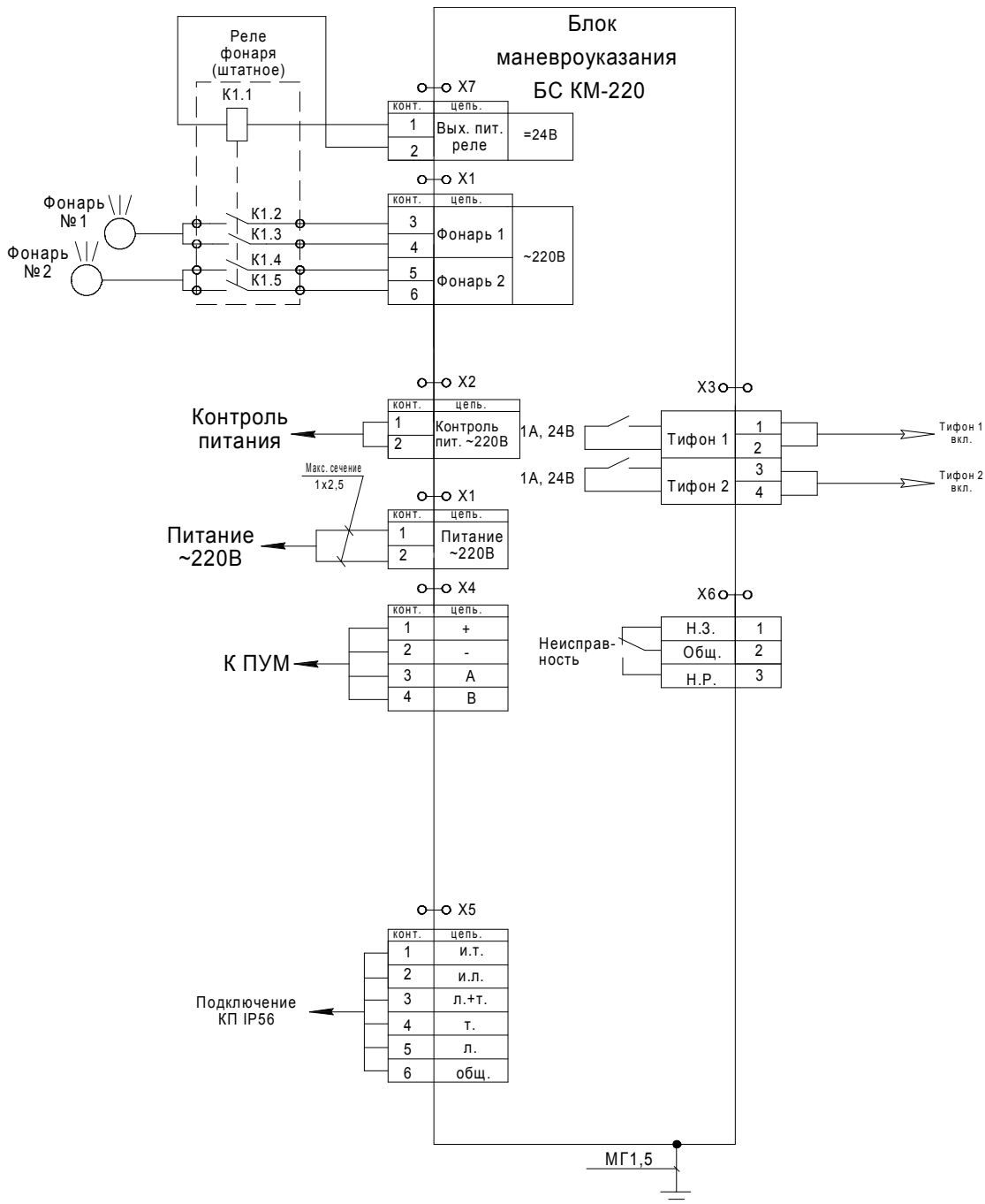
Блок силовой фонаря маневроуказания БС КМ-220 Схема электрическая подключений
