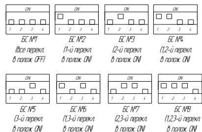
Варианты выставление DIP переключ. на силовом блоке BS KF-6 от 1 до 6 блока в системе:
