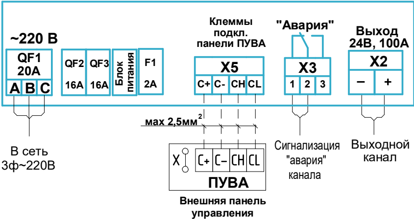
Подключение выходных кабелей
