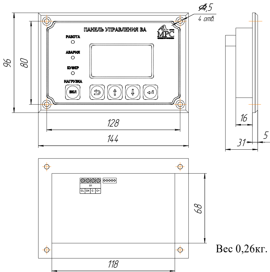
Панель управления ПУВА Габаритно-установочные размеры
