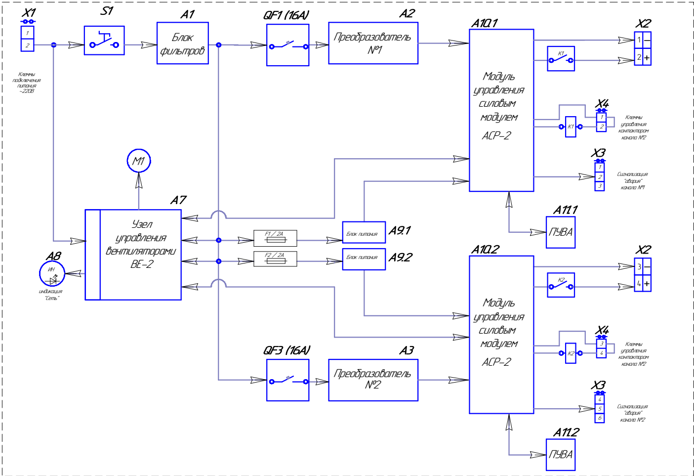
Схема структурная Агрегат ВА2450/50С
