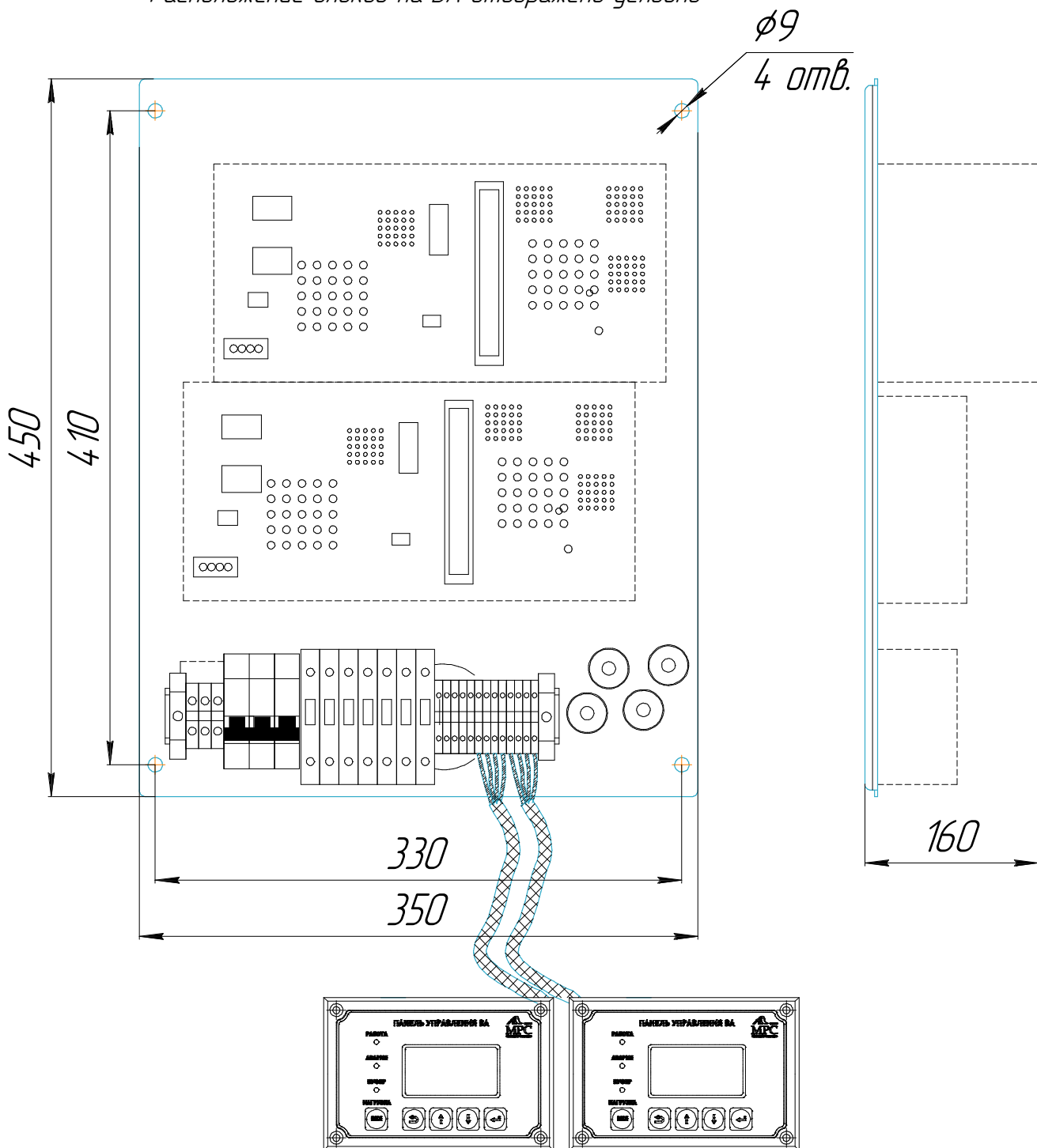
Агрегат ВАТ2435/35-01 IP20 Габаритно-установочные размеры
